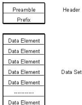
Figur 5.7.1 DICOM-protokolstruktur
